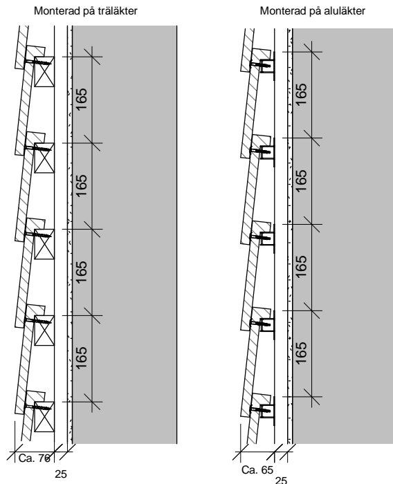
Opstalt 1:10
